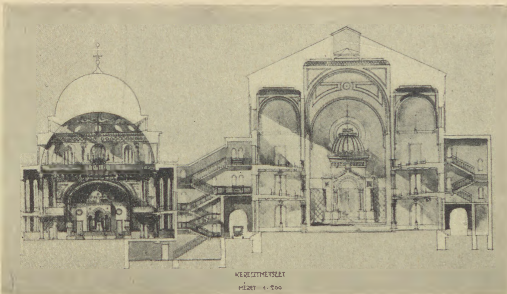
A pesti izr. hitközség számára építendő Kulturház és Iskola pályaterve. Komor Marcel és Komor János terve Preisgekrönter Plan von M. Komor und J. Komor
