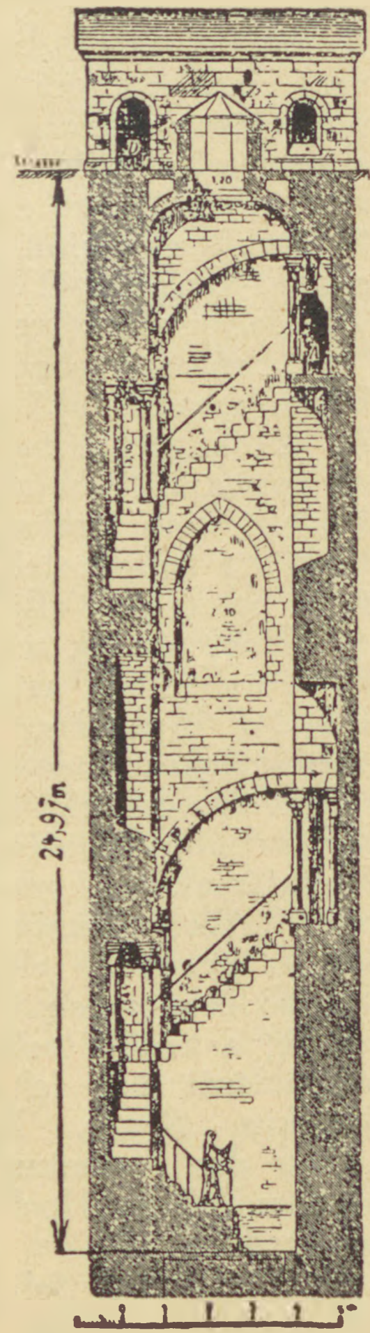
A friedbergi régi rituális fürdő keresztmetszete. (25 m.-nyire a föld alatt van a víz.)
