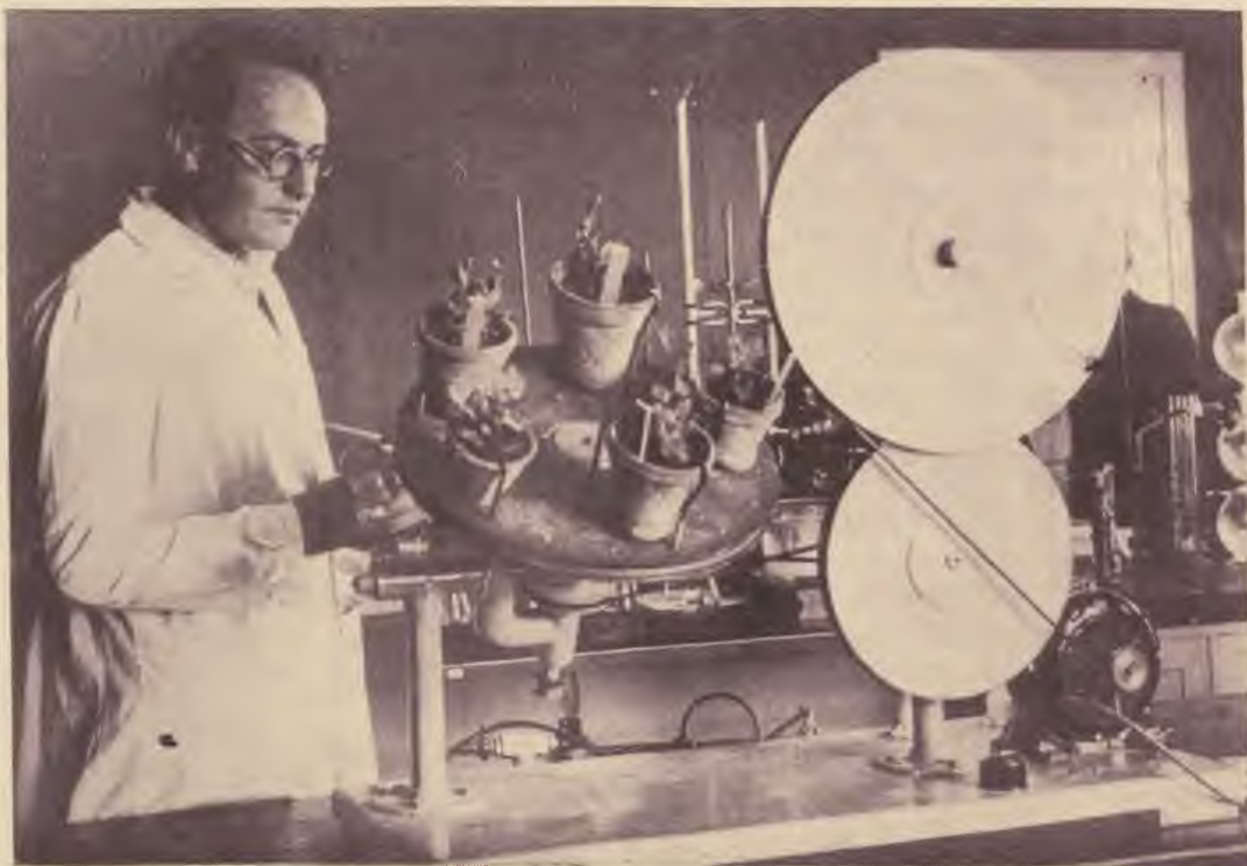
A botanikai osztály. Növényfiziológiai (klinostat) készülék a nehézségi erő befolyásának mérésére a növény fejlődésére vonatkozólag
